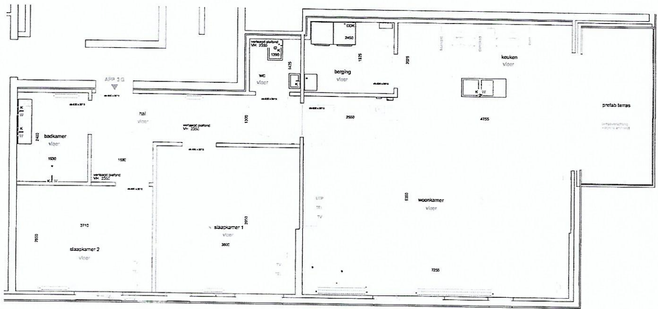
PLAN ALGEMEEN (1:50)
